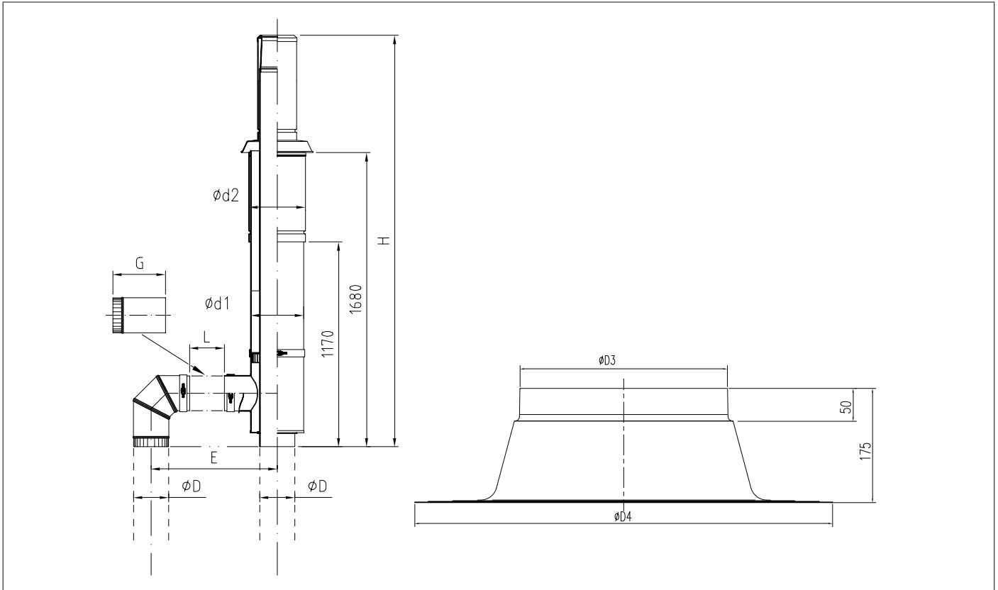
afb. 09 Verticale dakdoorvoer en plakplaat t.b.v. de Remeha Gas 310 ECO in gesloten uitvoering
